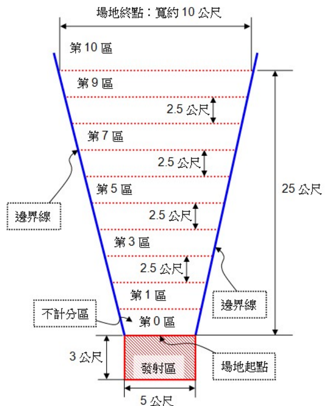
圖二 飛行競賽場地規劃示意圖
