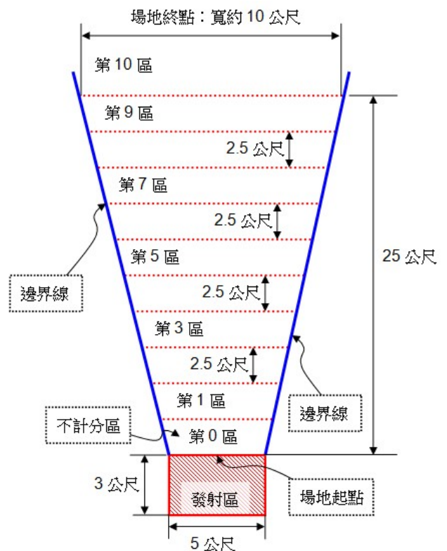
圖四 飛行競賽場地規劃示意圖
